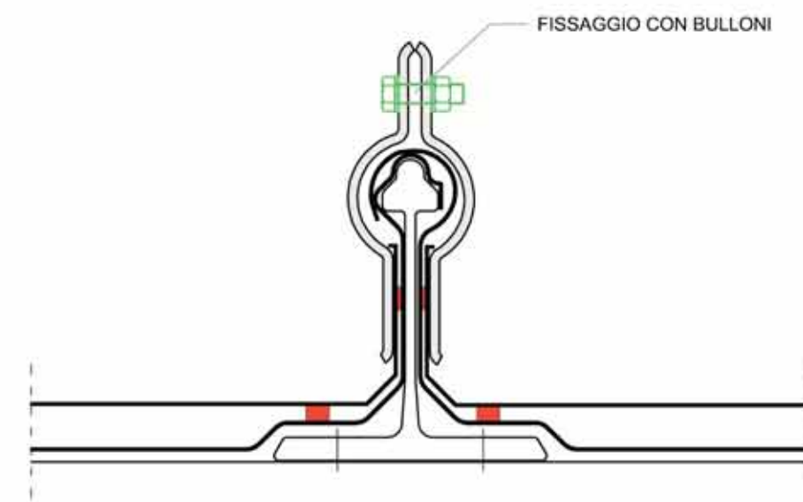
DETTAGLIO AGGRAFFATURA
